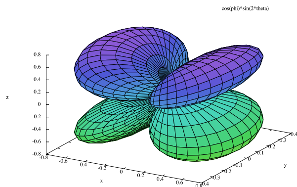
Maxima
