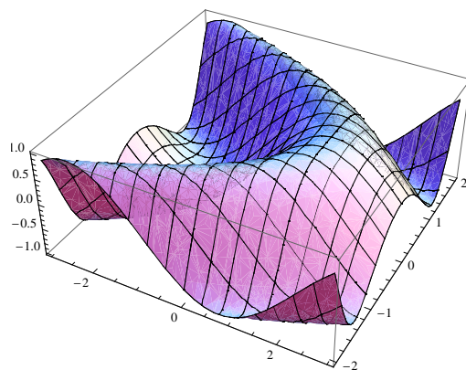
Mathematica
